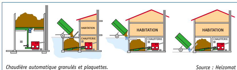
Chaudière automatique granulés et plaquettes.
